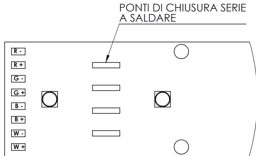
DETTAGLIO B SCALA 2 : 1
