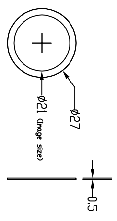
Gobos size (metal gobos)
