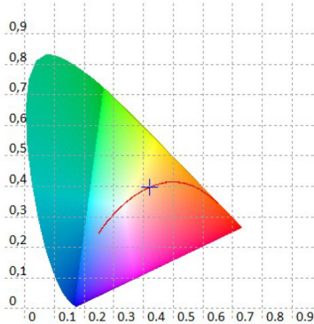
CIE 1931
