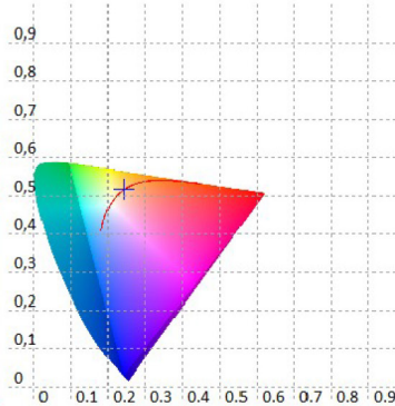
CIE 1976
