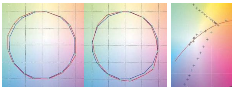
TM-30 Vectorgrafik bei 3200K und 5600K. Man erkennt bei beiden Grafiken, dass fast alle Farben gleichmäßig übersättigt wiedergegeben werden, bei 5600K ist jedoch eine stärkere Verschiebung ins Magenta zu erkennen
