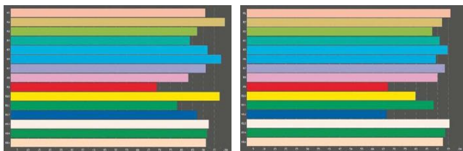
CRI-Farbanteile bei 3200K und 5600K, die übliche Rotschwäche von LED-Strahlern ist hier nicht ganz so ausgeprägt
